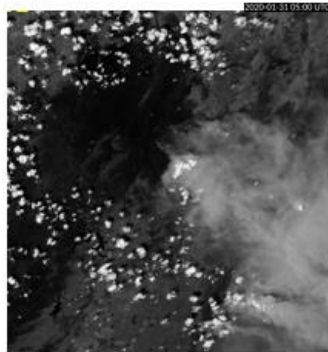
GEO-KOMPSAT-2A Band 3 (0.64 micron)
